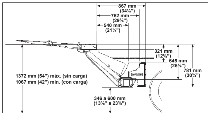
Dimensiones y requisitos de montaje del liftgate TE-25/TE-30
