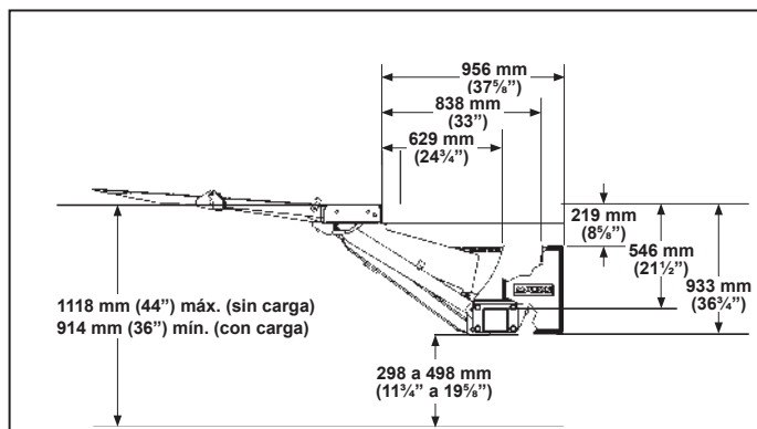
Dimensiones y requisitos de montaje del liftgate TE-25L/TE-30L
